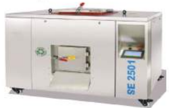
SE 2501 Capacity - 200Kgs
